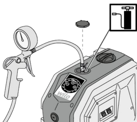
Fig. 7: Напълнете разширителния мембранен съд
